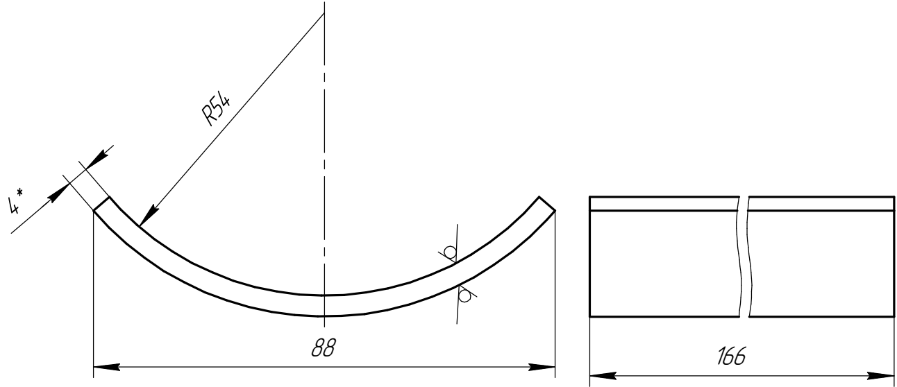
Дет. поз. 3
